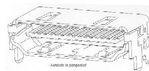
Aanzicht in perspectief
