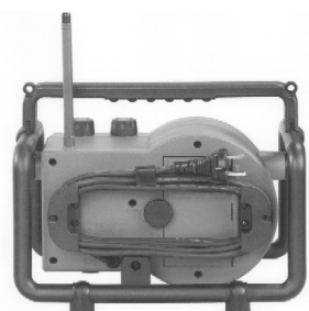
Achteraanzicht
