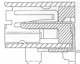
Doorsnede
